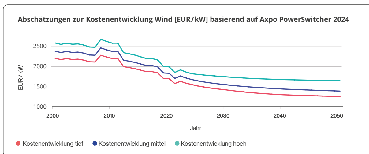
Abbildung 2: Die durchschnittlichen Kosten pro kW installierter Kapazität sind bei Wind in Deutschland in den letzten Jahrzehnten erheblich gefallen. Daten: real bei 2024-Werten, 1990–2023 historische Daten DE (umgelegt auf Preisniveau CH), 2024–2050 angenommene Entwicklung CH. Quelle: Axpo Power Switcher.
