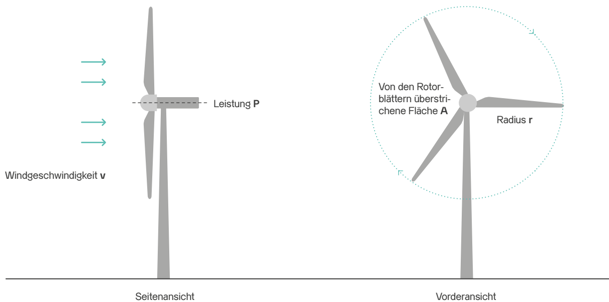
Abbildung 3: Vereinfachte Grafik einer Windturbine mit Radius der Rotorblätter «r», Windfangfläche «A», Windgeschwindigkeit «v» und Turbinenleistung «P».
