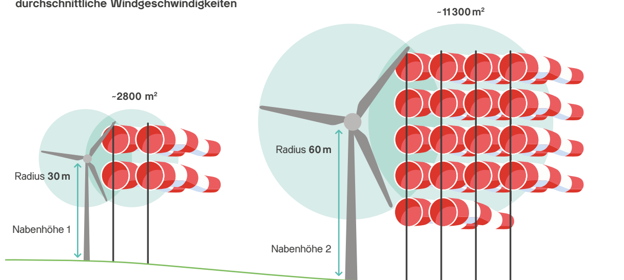
Abbildung 4: Eine Turbine mit zweimal so grossen Rotorblättern produziert rein aufgrund der grösseren von den Rotorblättern überstrichenen Fläche viermal mehr Windenergie. Dank der stärkeren Winde aufgrund der höheren Nabenhöhe fällt der Faktor der erzeugten Windenergie sogar noch höher aus.
